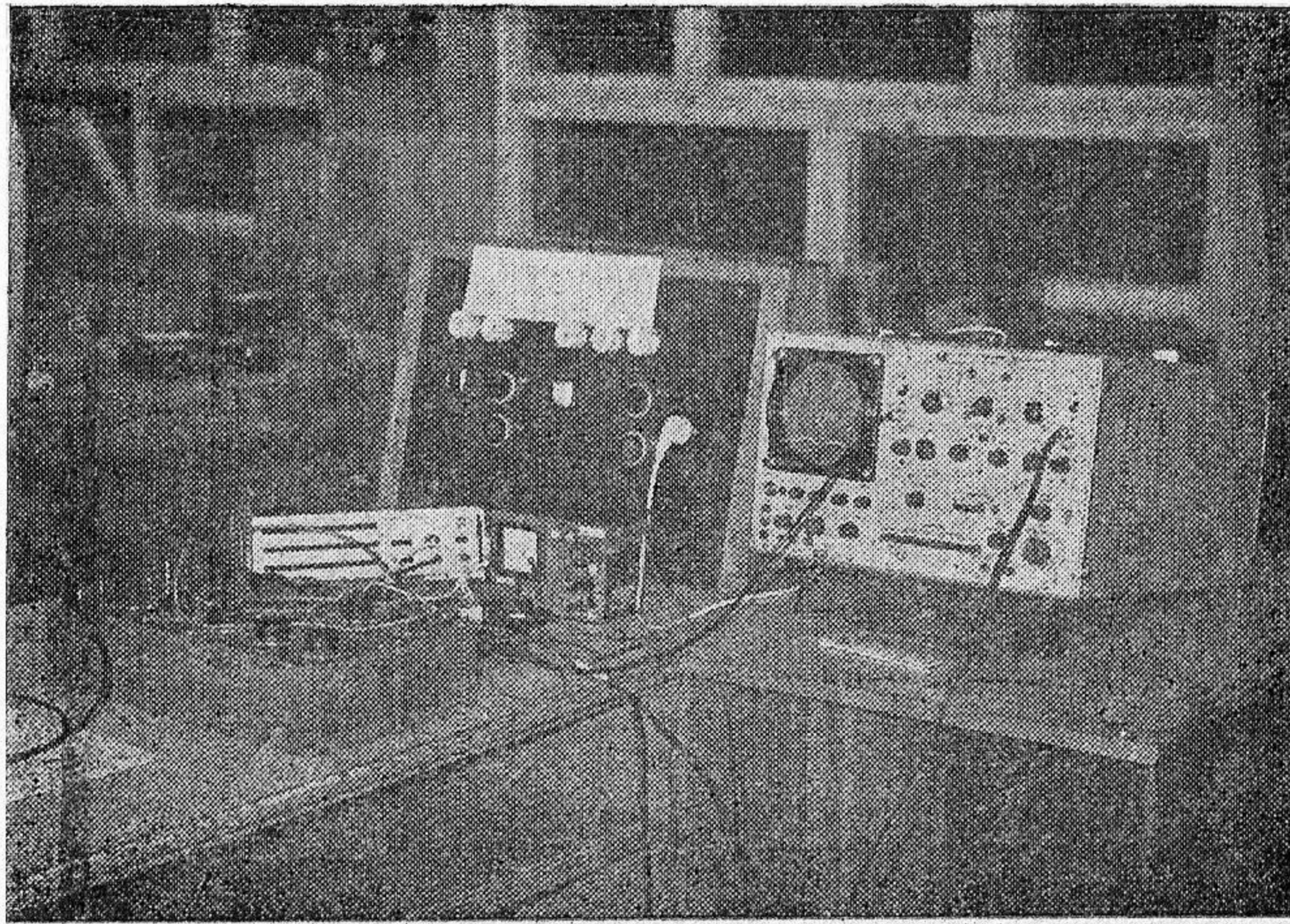
OLIMPIADA ELEKTRYCZNA STANOWISKO DO POMIARÓW WZMACNIACZY
